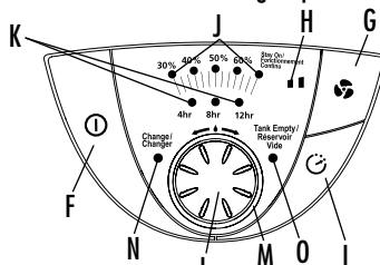
Figure 2 Panneau de Contrôle (gros plan)
